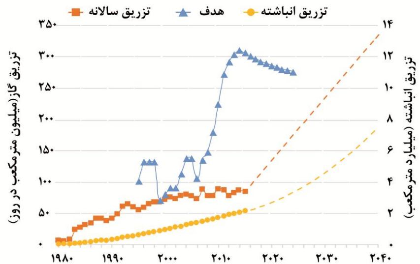
شکل ۴. داده‌های تاریخی و برآوردهای آتی از تزریق سالانه گاز و اهداف پیشین آن (محور سمت چپ)، و تزریق گاز انباشته (محور سمت راست) به مخازن نفت خام ایران.
